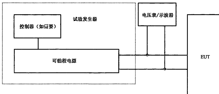
图 A.2 基于可编程电源的试验发生器示例
