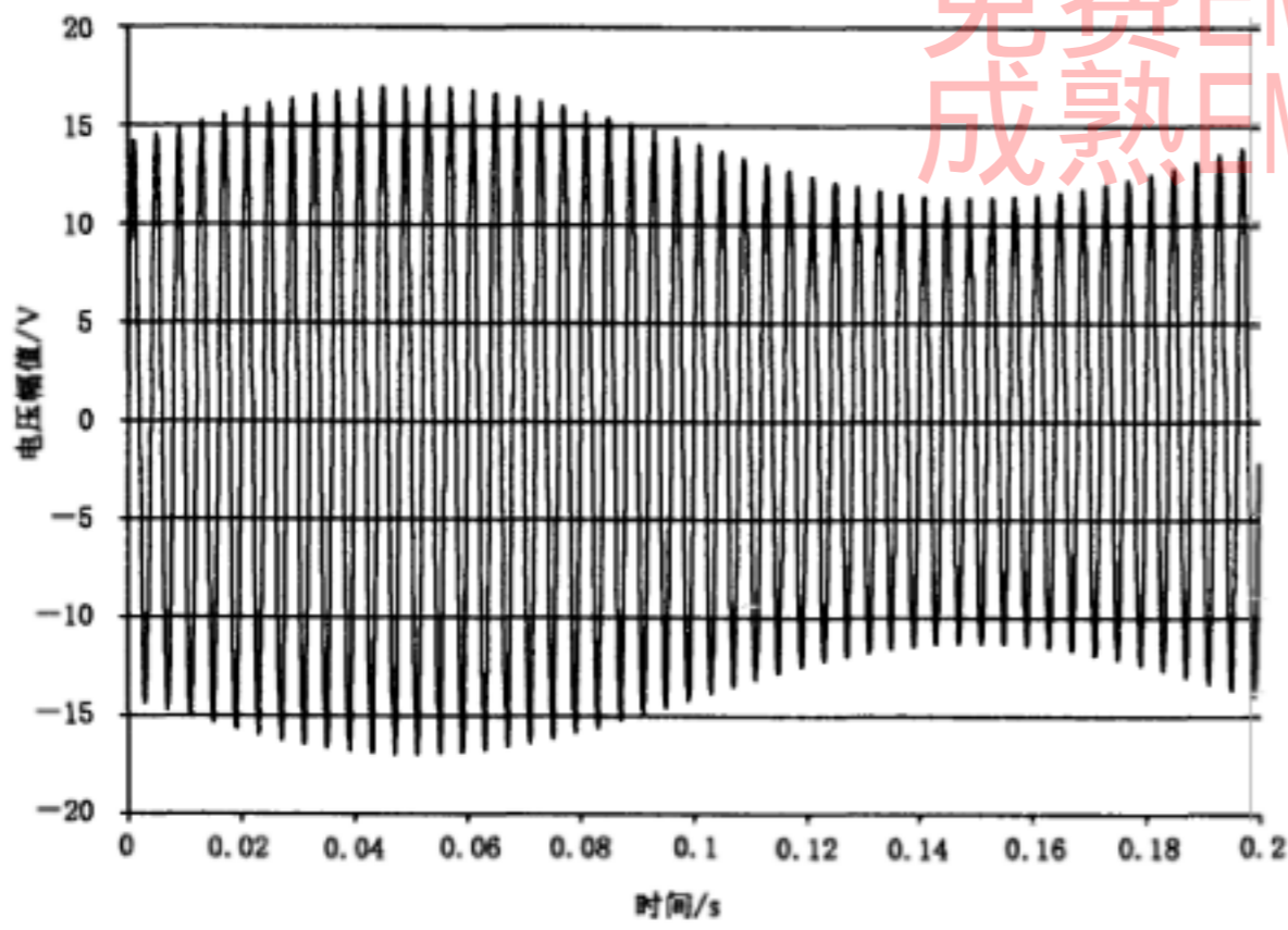
a) 有 20% 幅值波动的 5 次谐波
