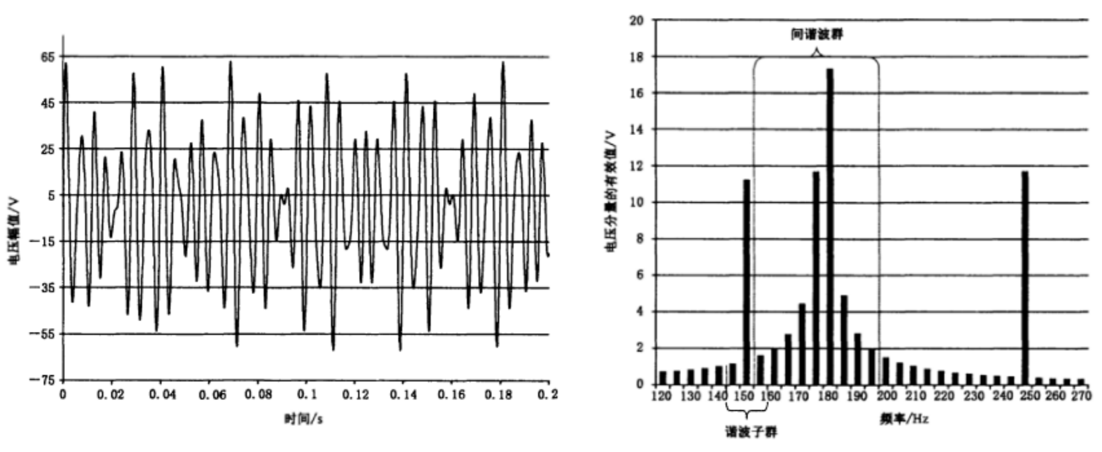
图 C.4 178 Hz 的通信信号以及 3 次、5 次谐波
