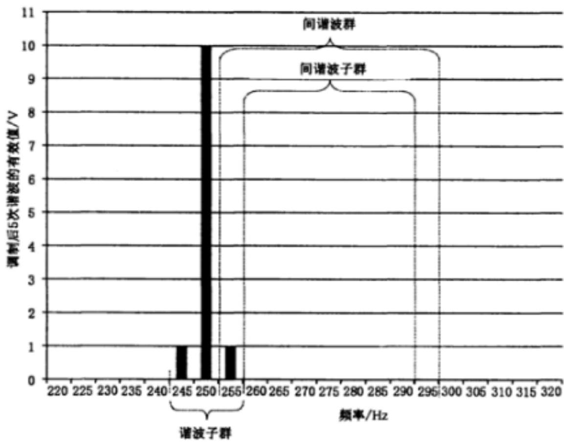
a) 有 20% 幅值波动的 5 次谐波
