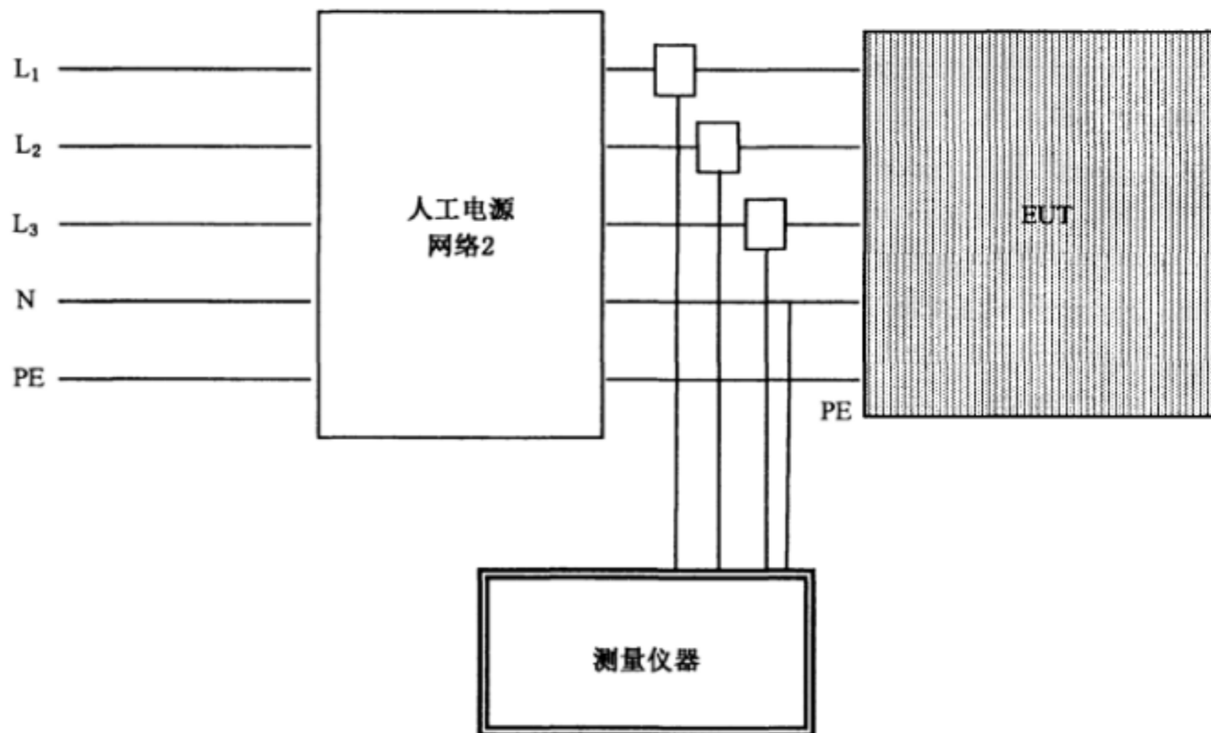
b) 三相测量布置
