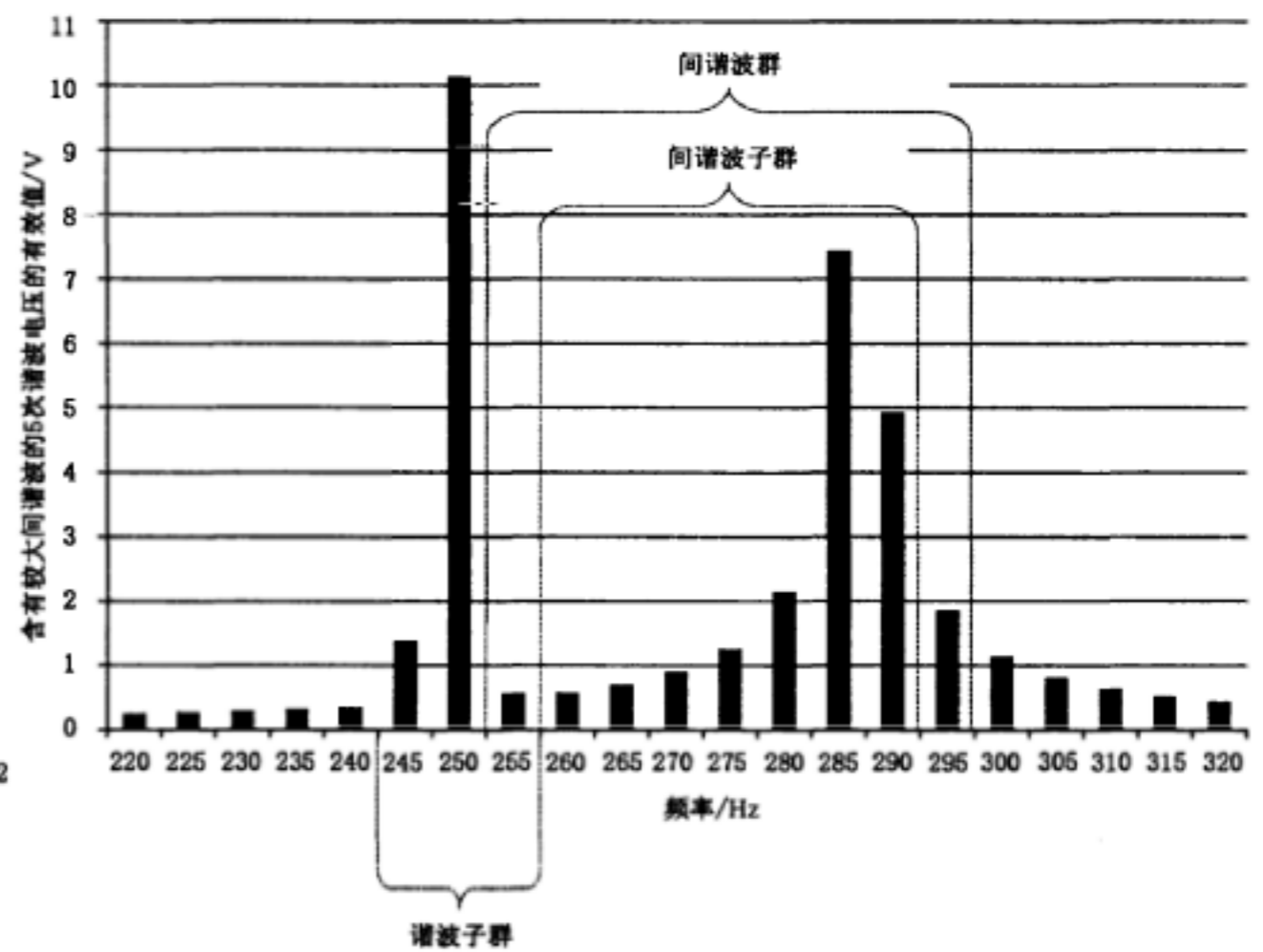
f) 频谱: 信号的总和
