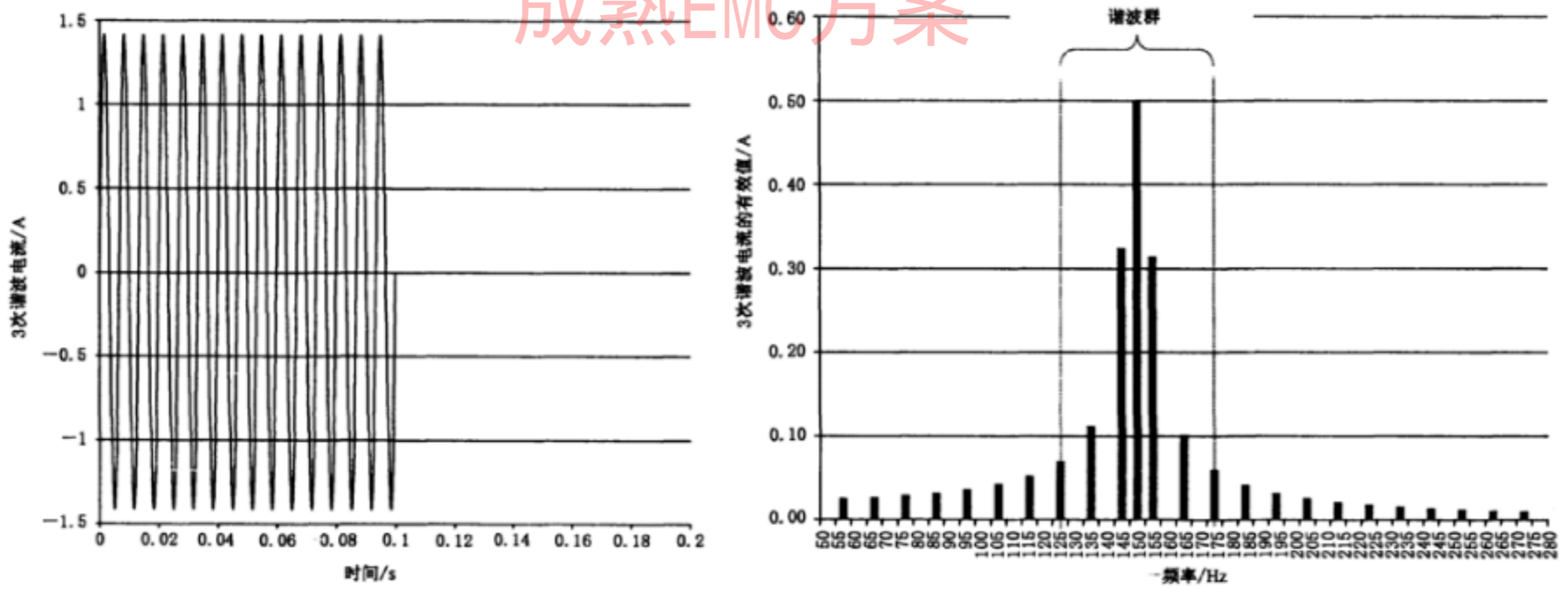
图 C.3 某微波器具波动的 3 次谐波电流
