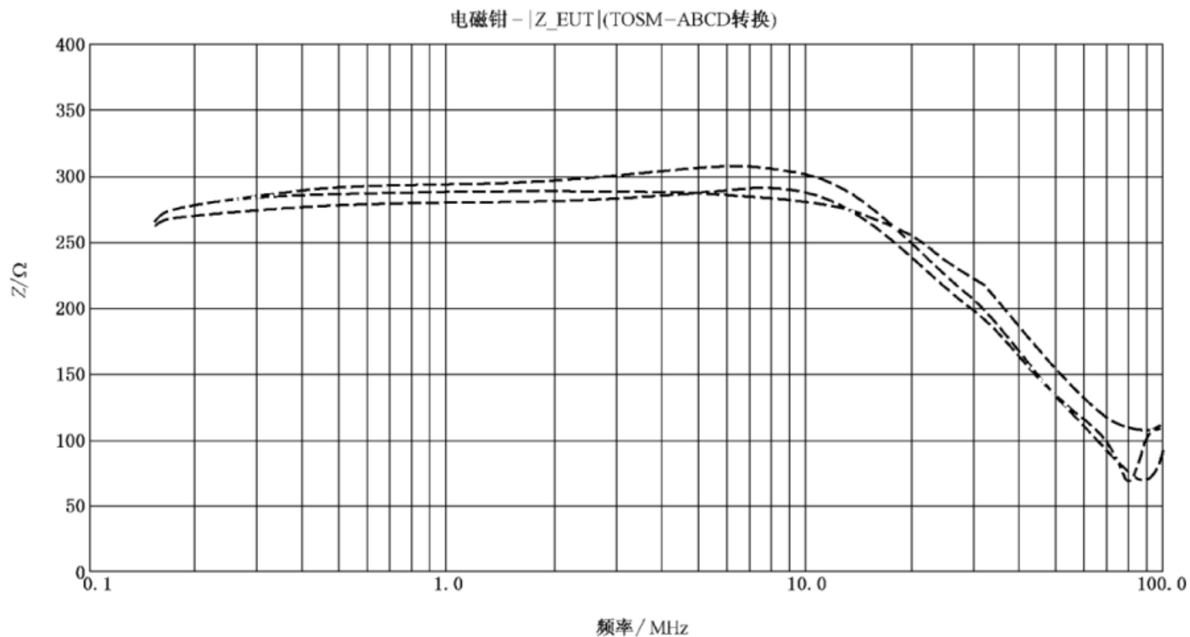
图 A.7 三种电磁钳阻抗的典型实例
