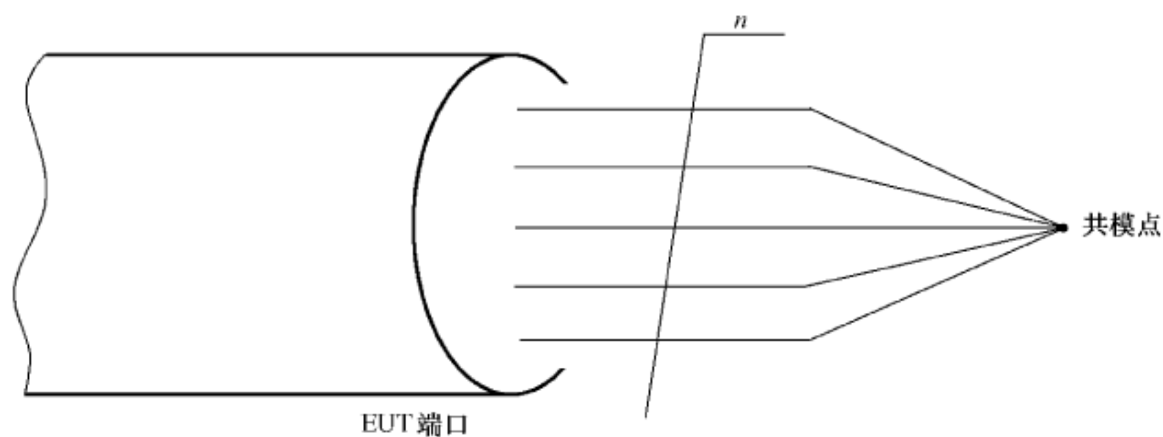
a) 非屏蔽电缆的共模点定义
