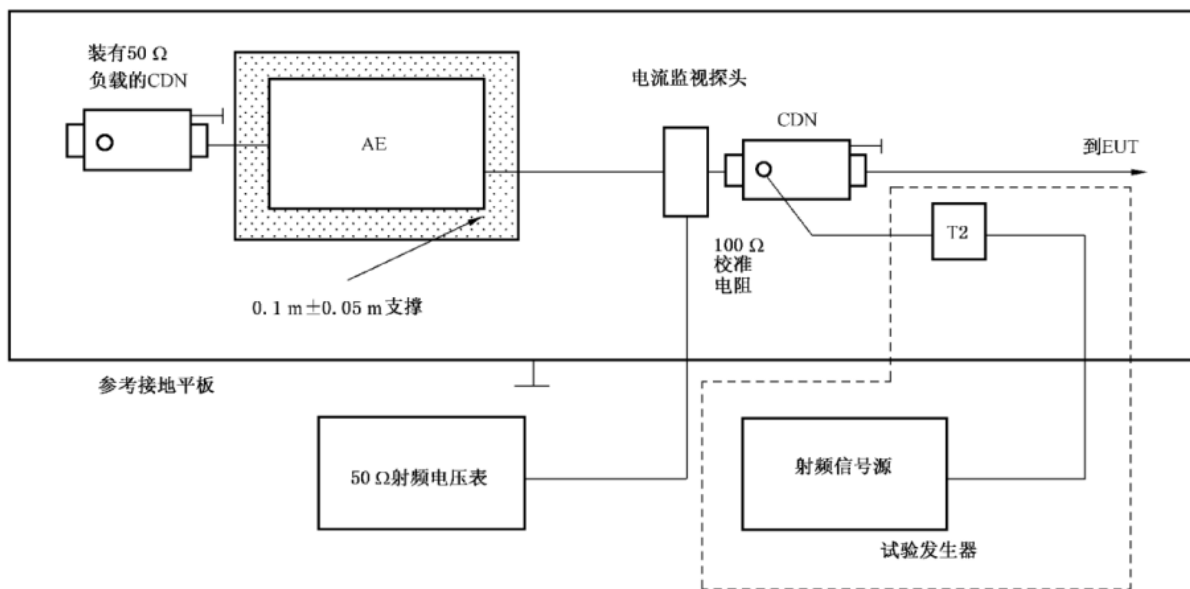
图 H.2 使用电流探头测量阻抗
