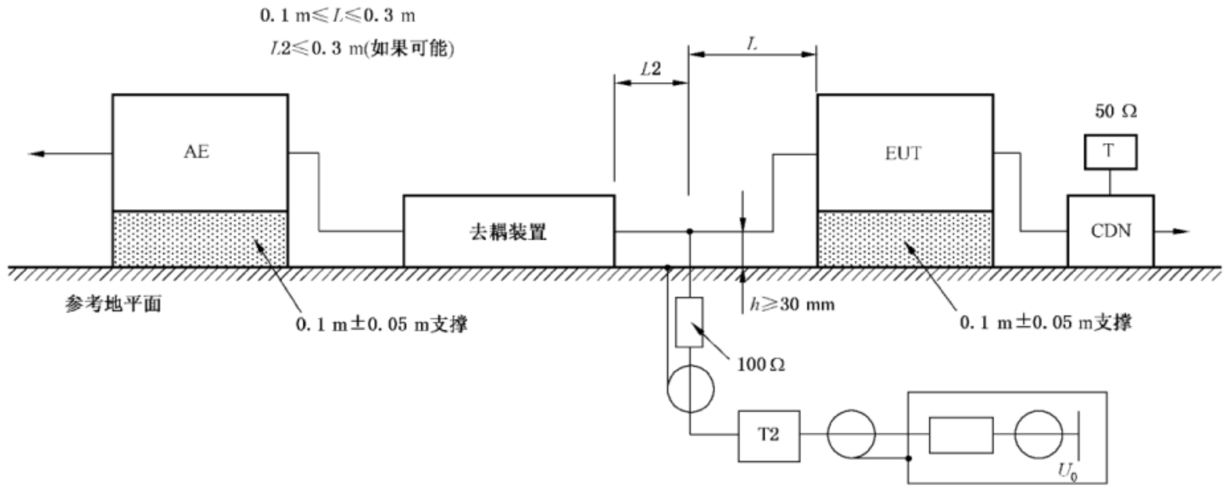
b) 直接注入到屏蔽电缆的原理图
