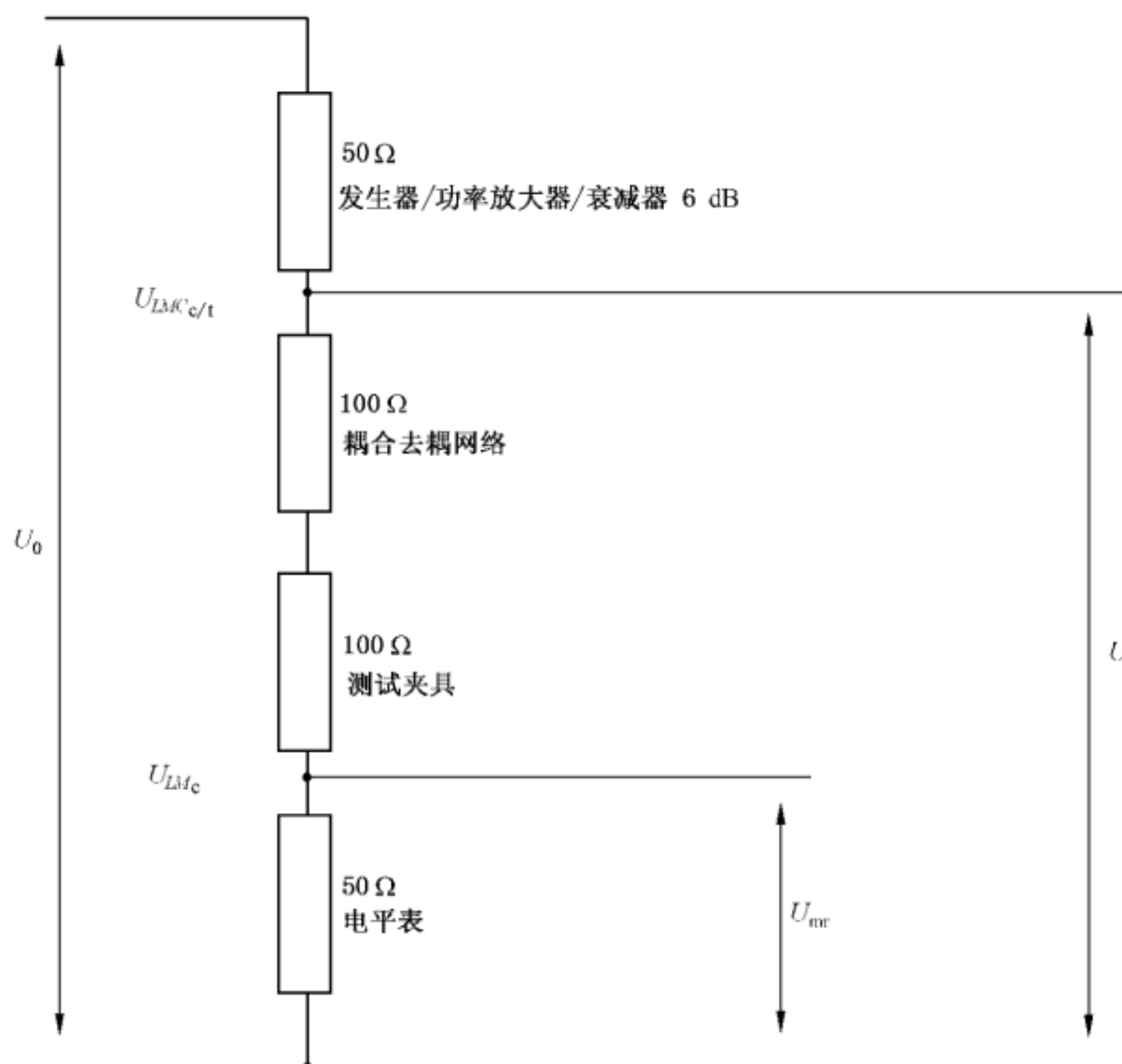
图 G.5 电平调整电路示意图
