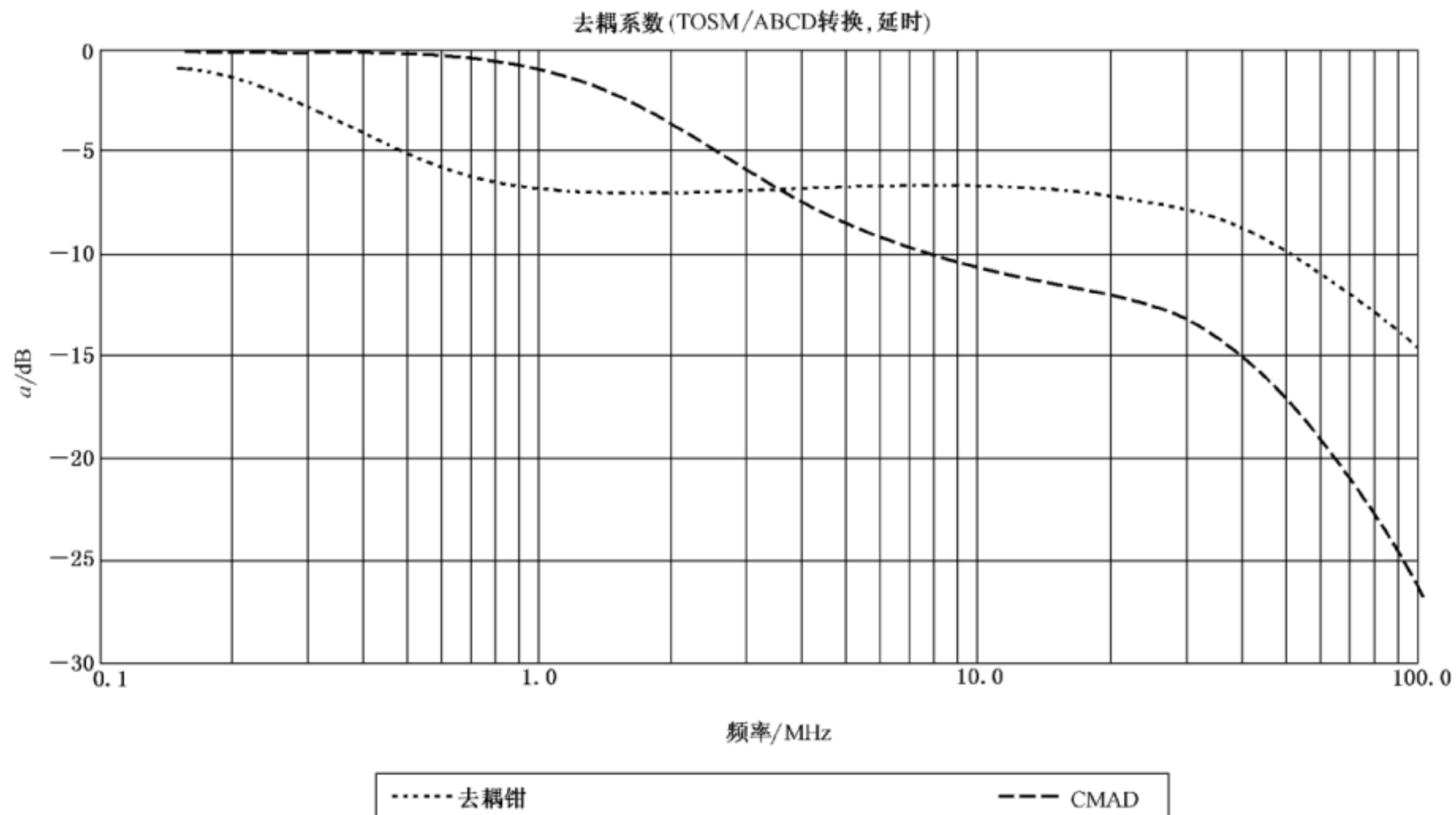
图 A.14 去耦系数的典型实例
