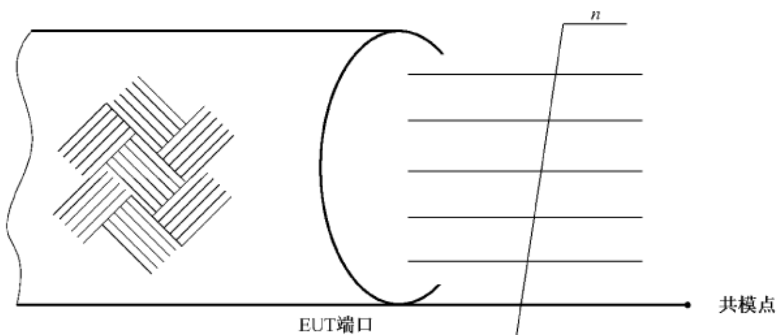
b) 屏蔽电缆的共模点定义
