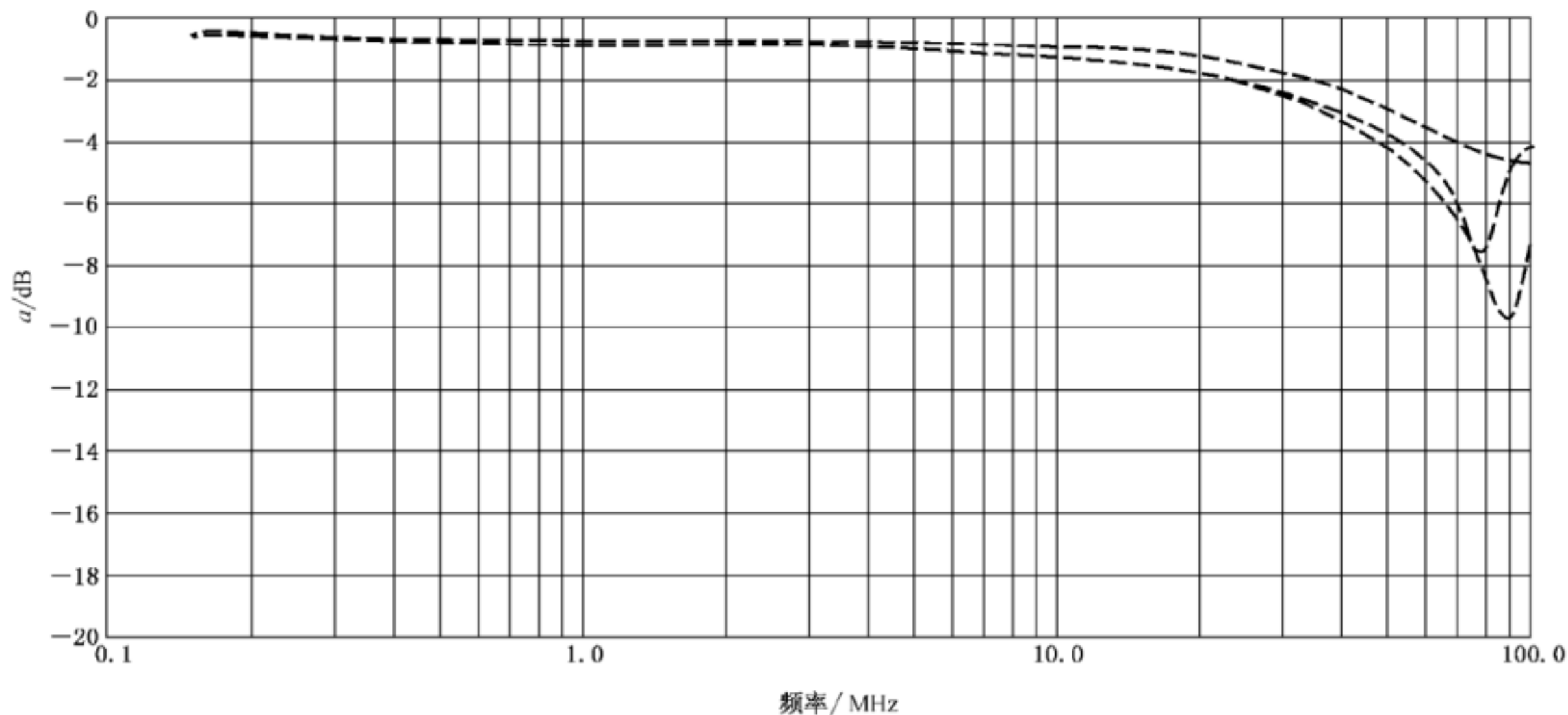
图 A.8 3 种电磁钳去耦系数的典型实例
