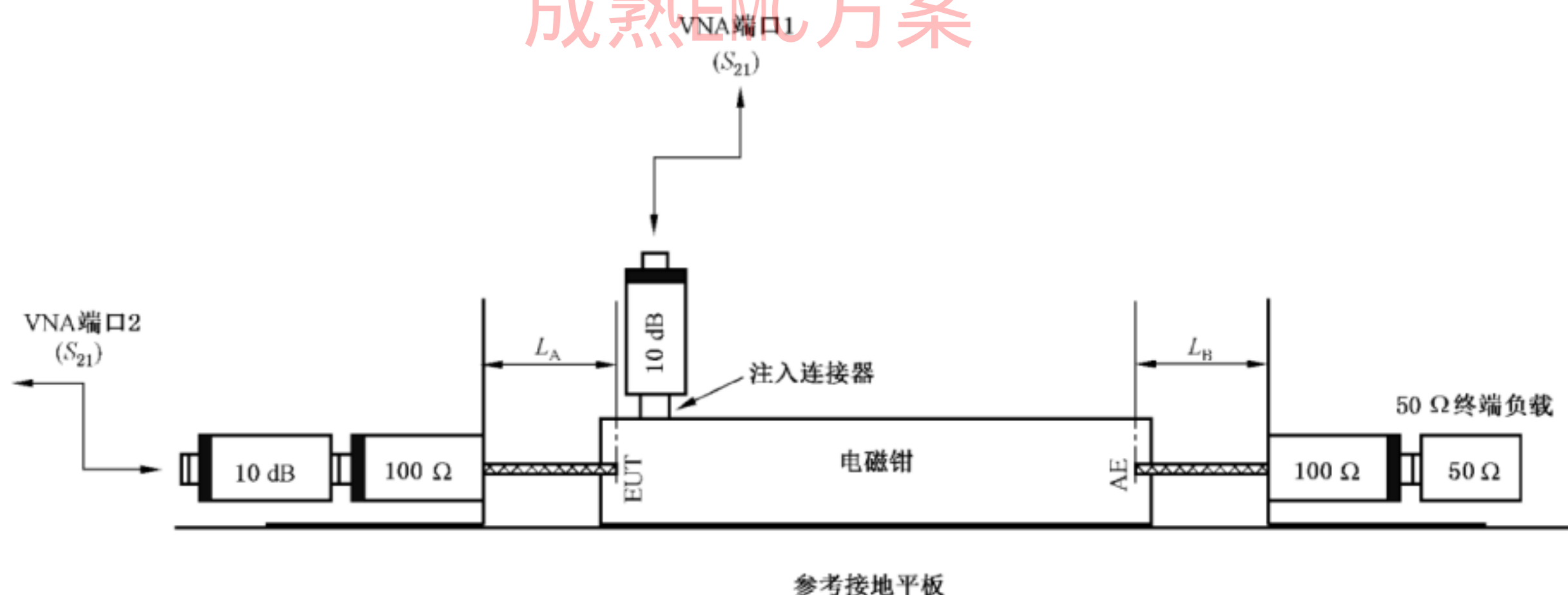
图 A.10 S_{21} 耦合系数测量布置
