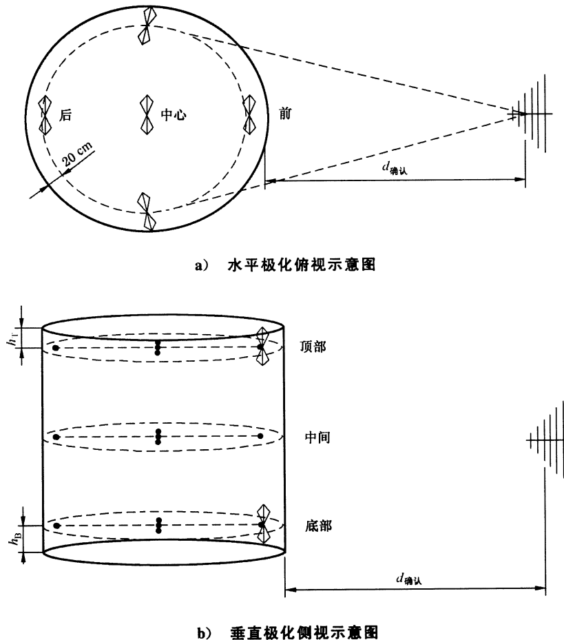
b) 垂直极化侧视示意图
