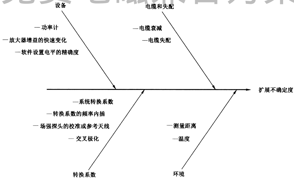
图 D.2 对抗扰度试验方法有影响因素示例
