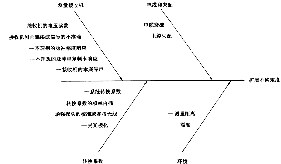
图 D.1 发射测量影响因素的例子
