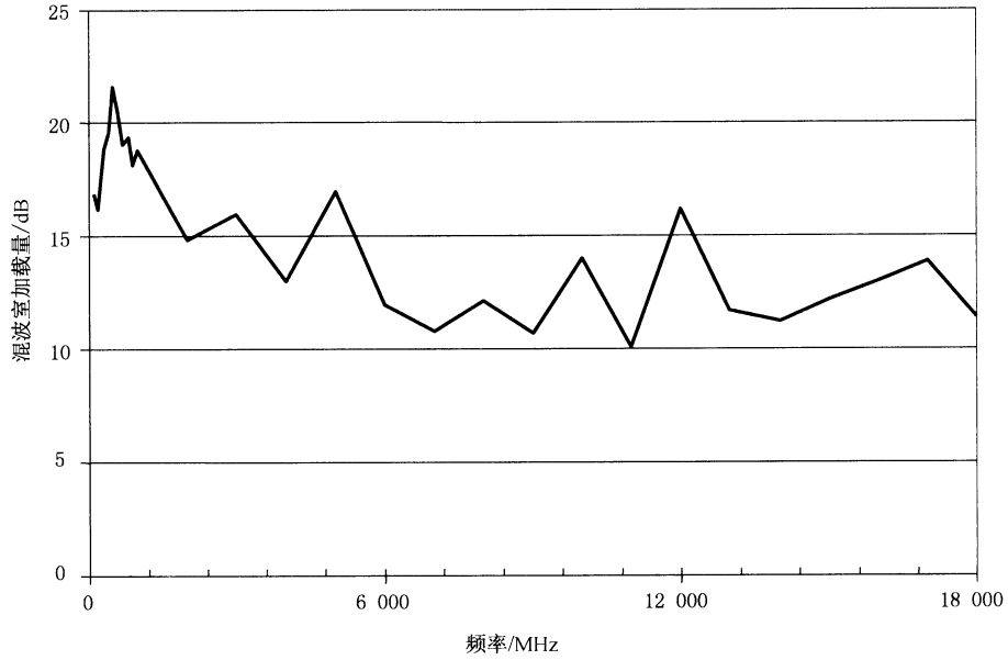
图 A.15 加载效应试验的加载量
