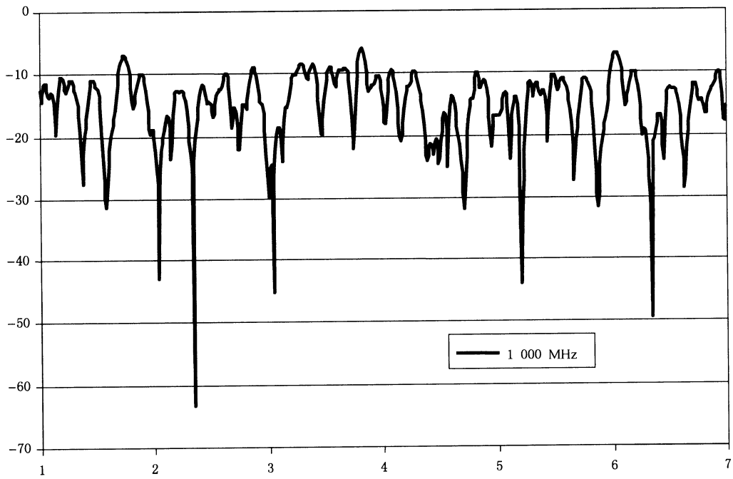
图 C.2 1 000 MHz 时,接收功率(dBm)与搅拌器转动(s)的关系
