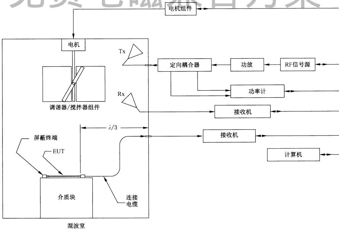
图 F.1 典型的试验布置
